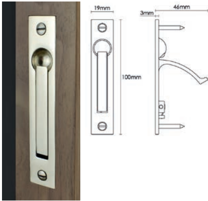
2600 Light Edge Pull
