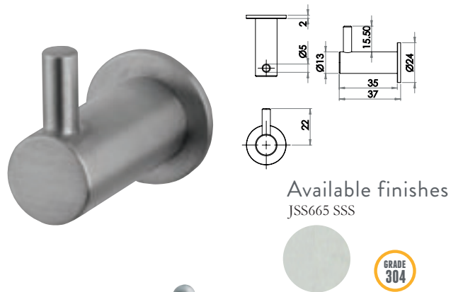
Robe Hook
